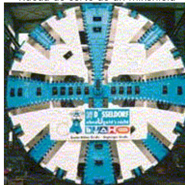
Rueda de corte de un mixshield
